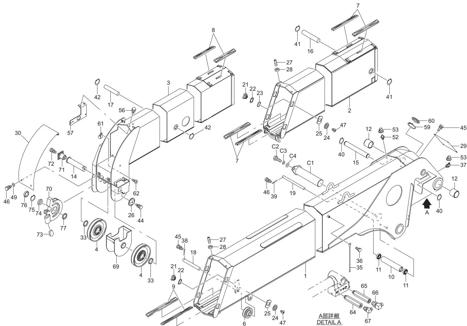
3 段ブーム組立 (URV503-1-GO) Fig.1-1 3-section BOOM ASS'Y(URV503-1-GO)
