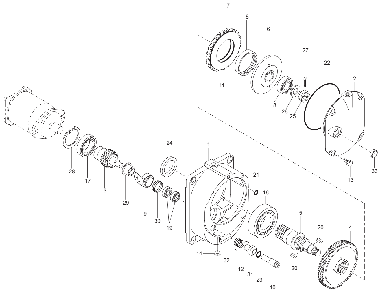
Fig. 10-1-1 ホイストウインチ減速機 ASS'Y (URV500-1-GO 系) HOIST WINCH REDUCTION GEAR ASS'Y (URV500-1-GO series)
