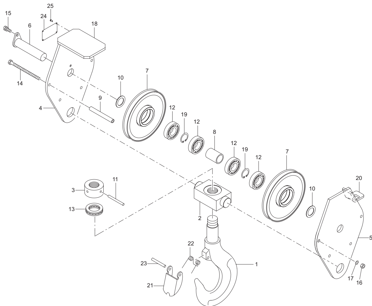
フック組立 (URV500-1-GO 系) Fig.3-2 HOOK ASS'Y (URV500-1-GO series)
