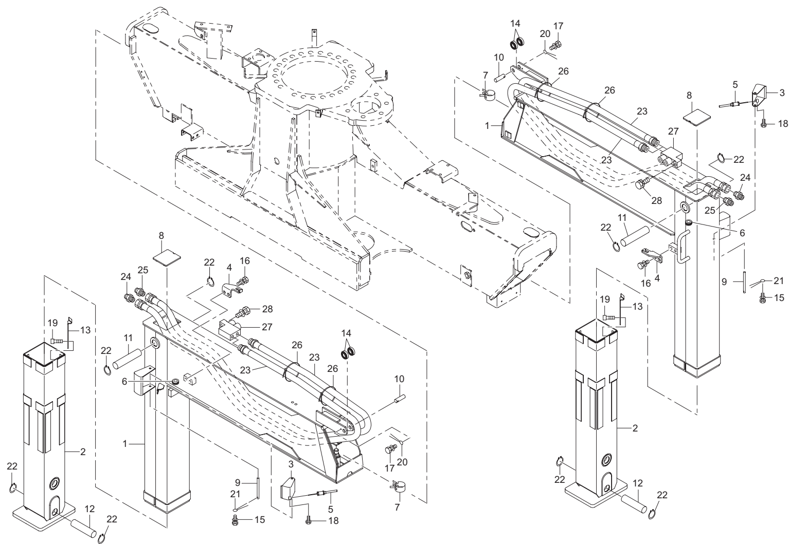
インナボックス組立 (URV500-1-GO 系) Fig. 8-1-1 INNER BOX ASS'Y (URV500-1-GO series)
