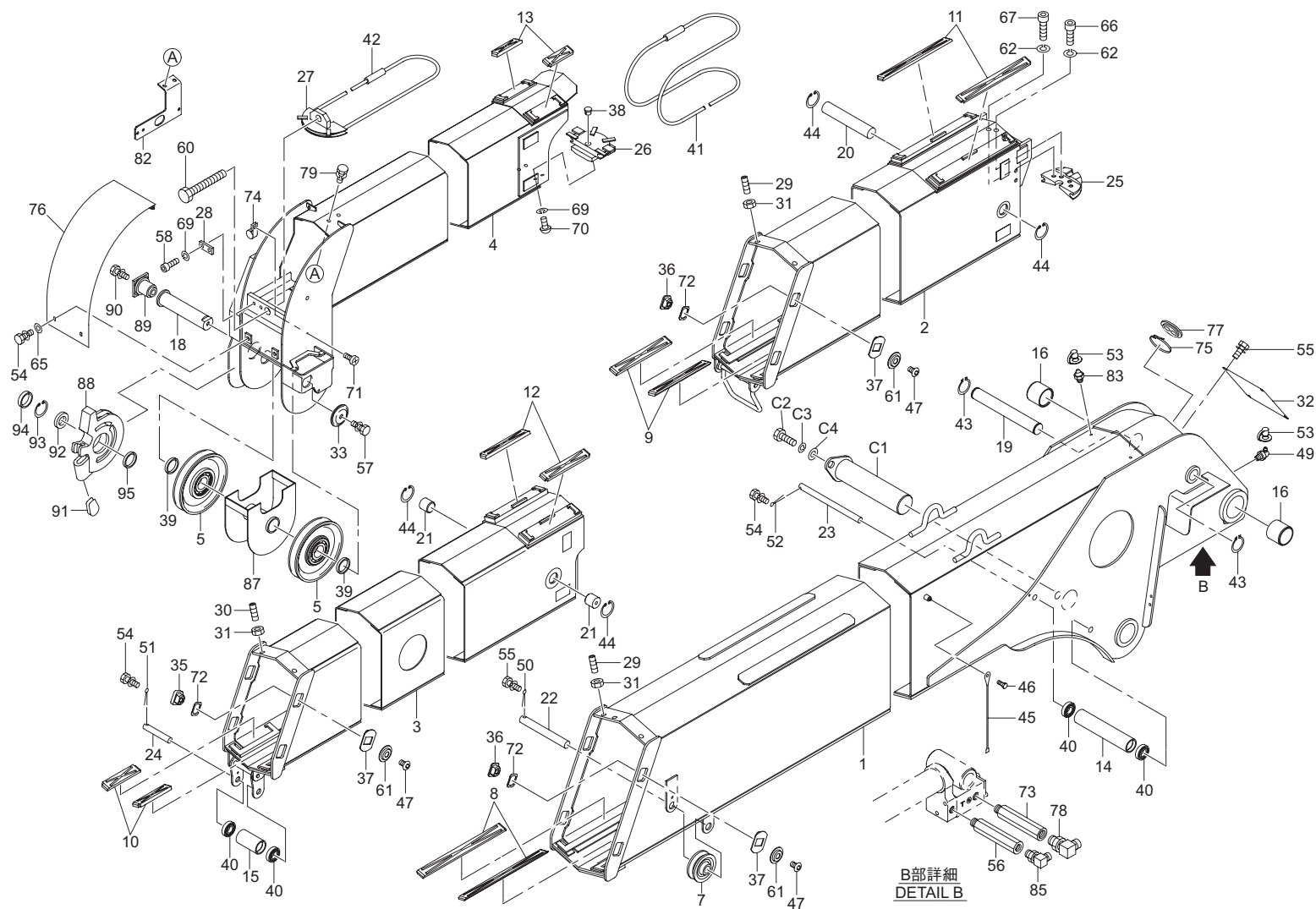
4 段ブーム組立 (URV504-1-GO) Fig.1-3 4-section BOOM ASS'Y(URV504-1-GO)
