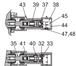
E 部詳細 DETAIL E
