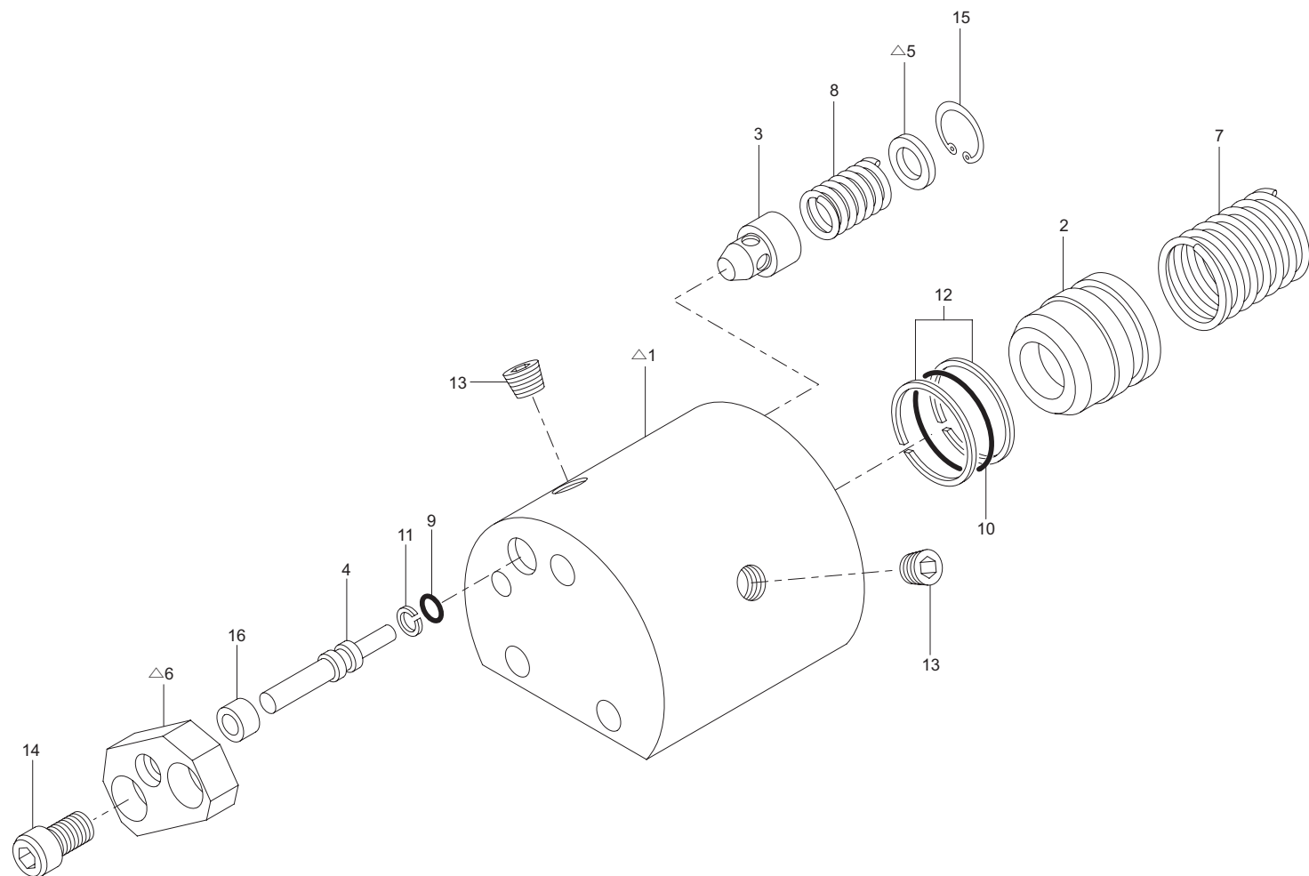
切換バルブ ASS'Y(URV504-1-GO) Fig. 2-3-1 SELECTOR VALVE ASS'Y(URV504-1-GO)
