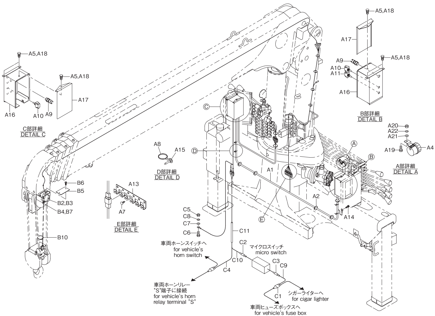
警報装置組立 (URV500-1-GO 系) Fig. 4-2 ALARM DEVICE ASS'Y (URV500-1-GO series)
