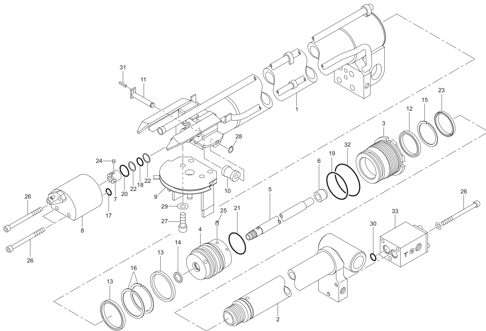
テレシリンダ (1) 組立 (URV504-1-GO) Fig. 2-3 SELECTOR VALVE ASS'Y(URV504-1-GO)
