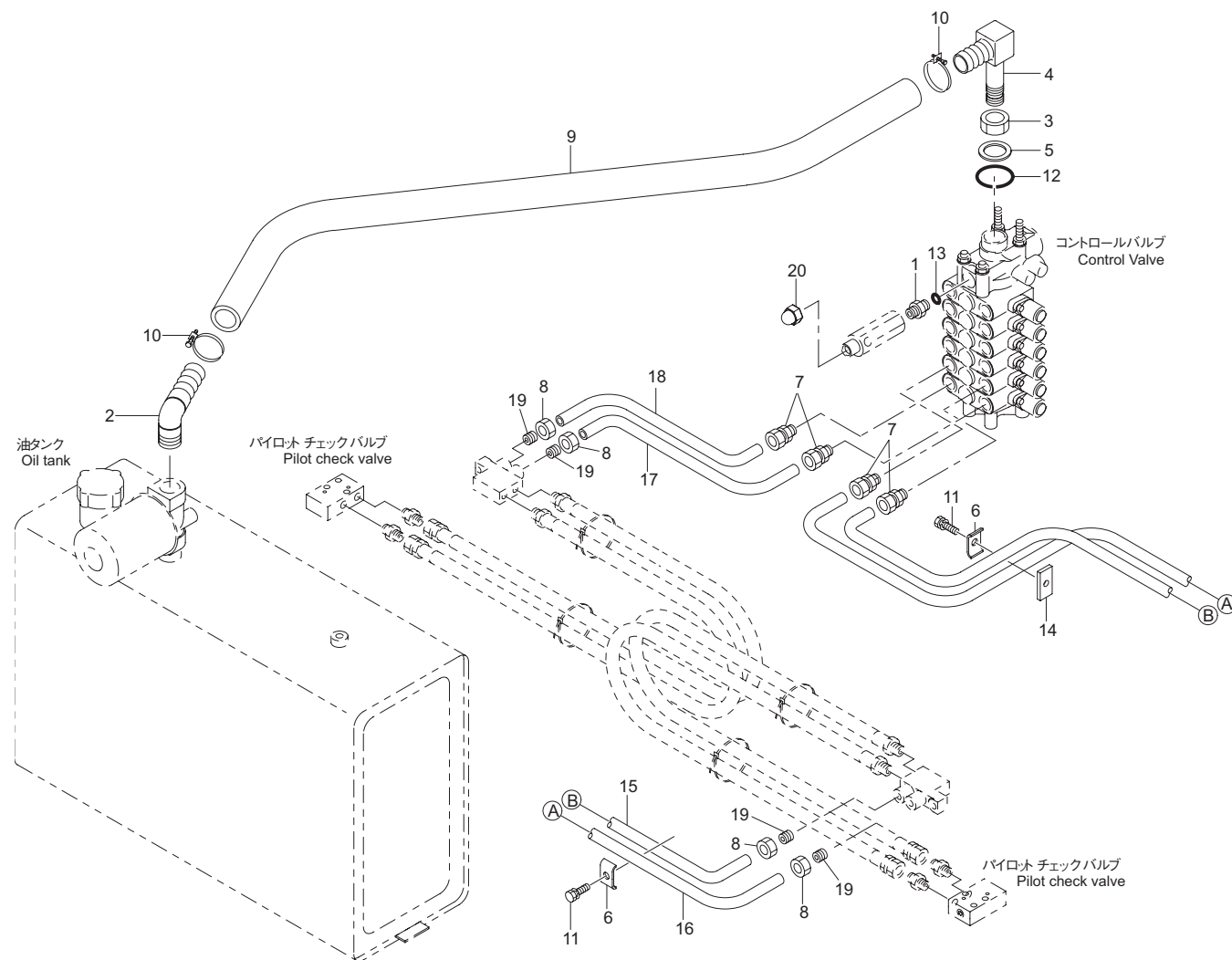
パイピング (アウトリガ) (URV500-1-GO 系) Fig. 6-2-5 PIPING(Outrigger) (URV500-1-GO series)
