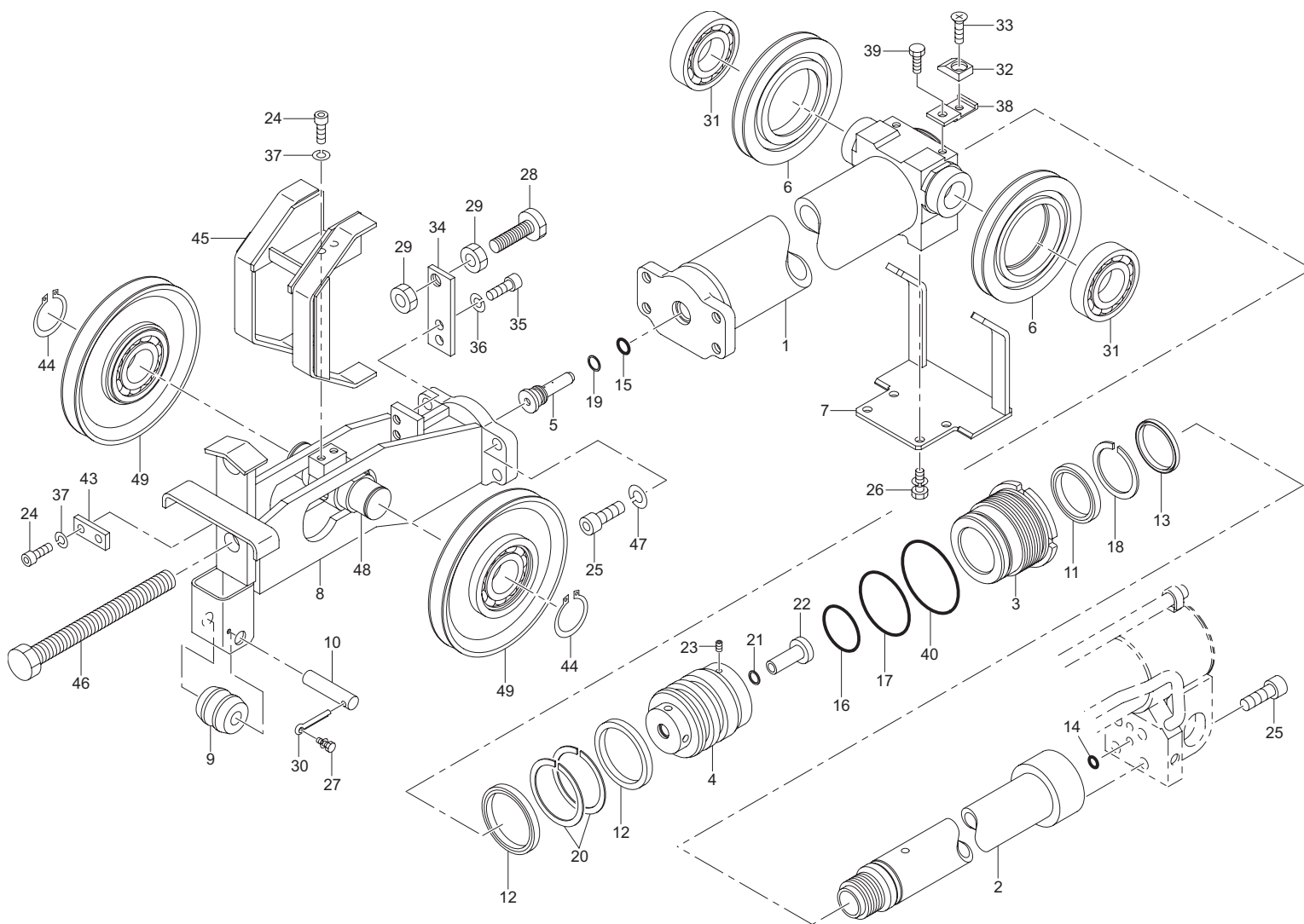
テレシリンダ (2) 組立 (URV504-1-GO) Fig. 2-4 TELESCOPE CYLINDER(2) ASS'Y(URV504-1-GO)
