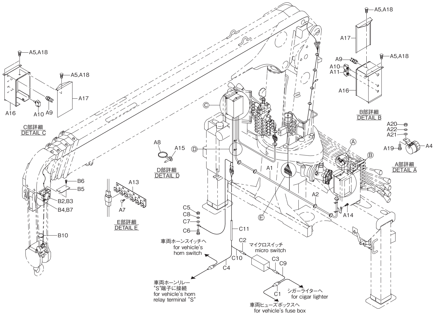
警報装置組立 (URV500-1-GO 系) Fig. 4-2 ALARM DEVICE ASS'Y (URV500-1-GO series)
