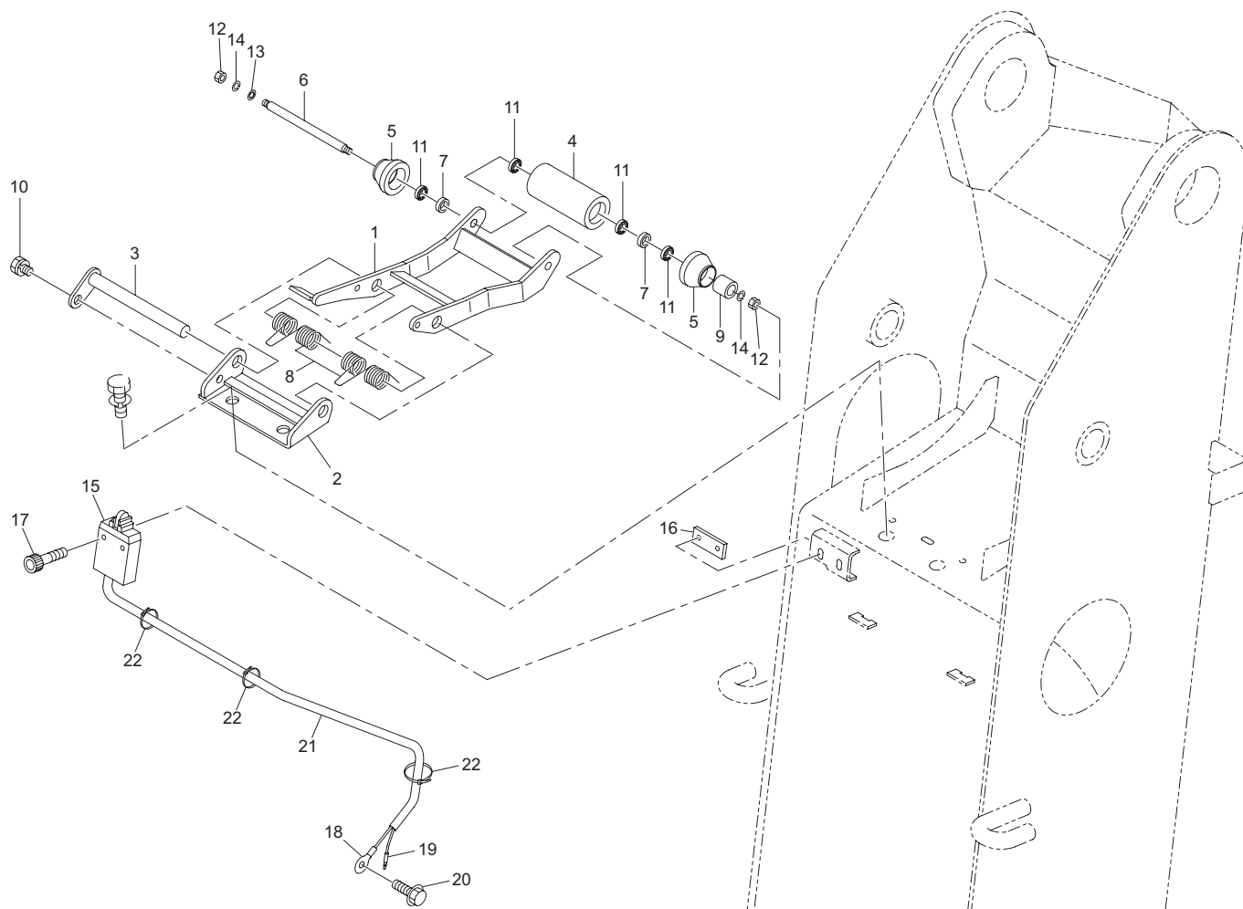
ワイヤロープ押えローラ装置組立 (URV500-1-GO 系) Fig. 19-1 WIRE ROPE CLAMPING ROLLER DEVICE ASS'Y (URV500-1-GO series)
