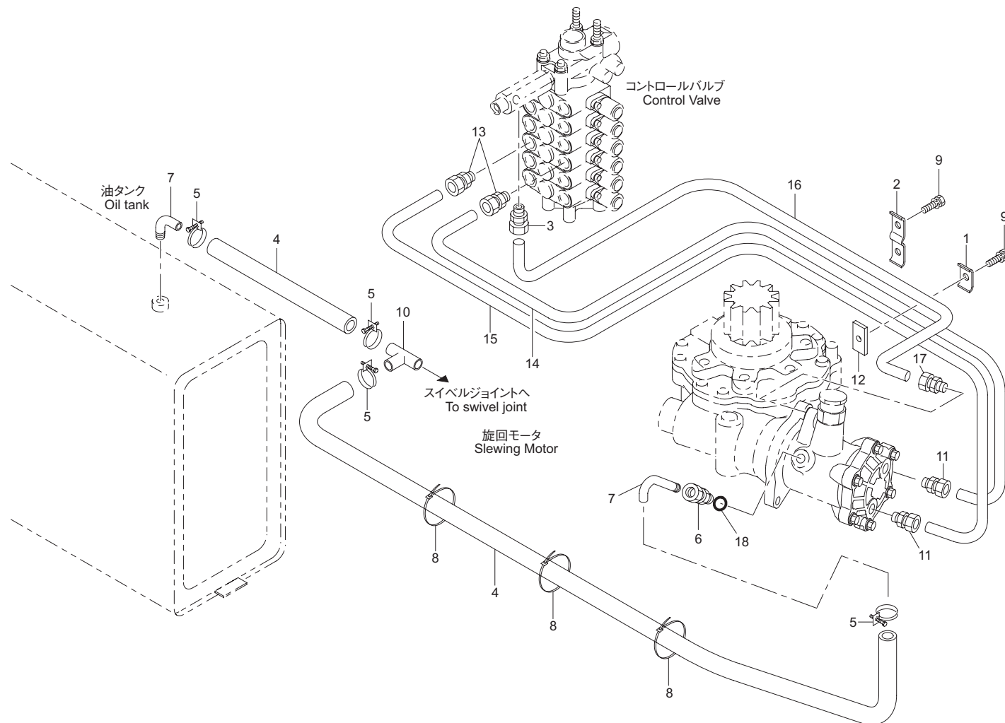
パイピング (旋回モータ) (URV500-1-GO 系) Fig. 6-2-4 PIPING(Slewing motor)(URV500-1-GO series)
