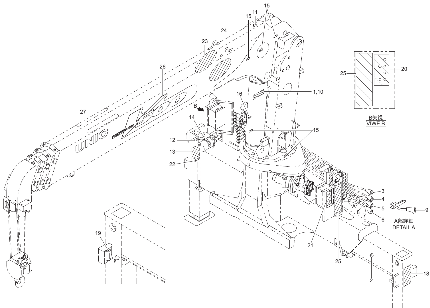
Fig. 16-2 銘板 (URV500-1-GO 系) NAME PLATE (URV500-1-GO series)
