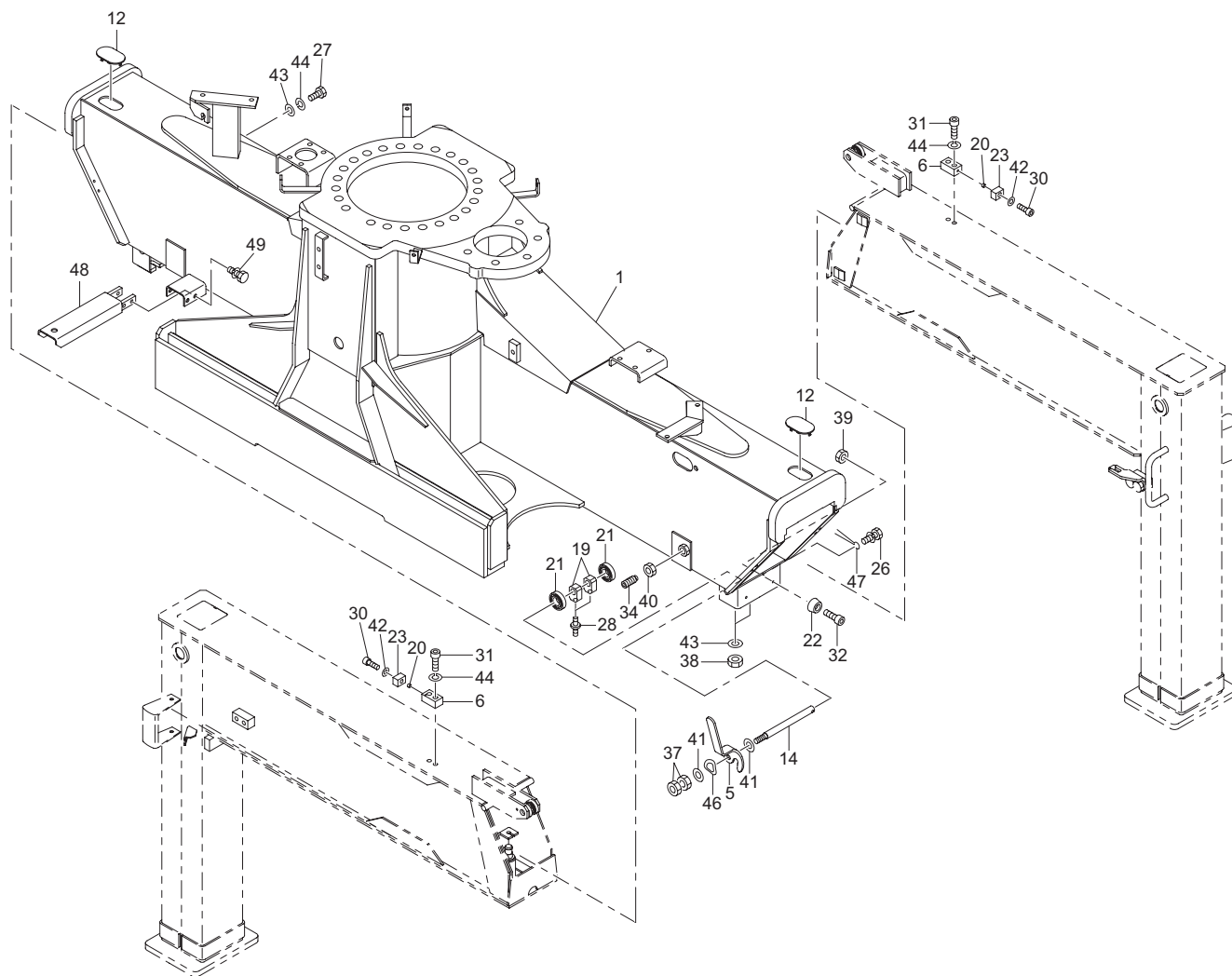
ベース組立 (URV500-1-GO 系) Fig. 8-1 BASE ASS'Y (URV500-1-GO series)
