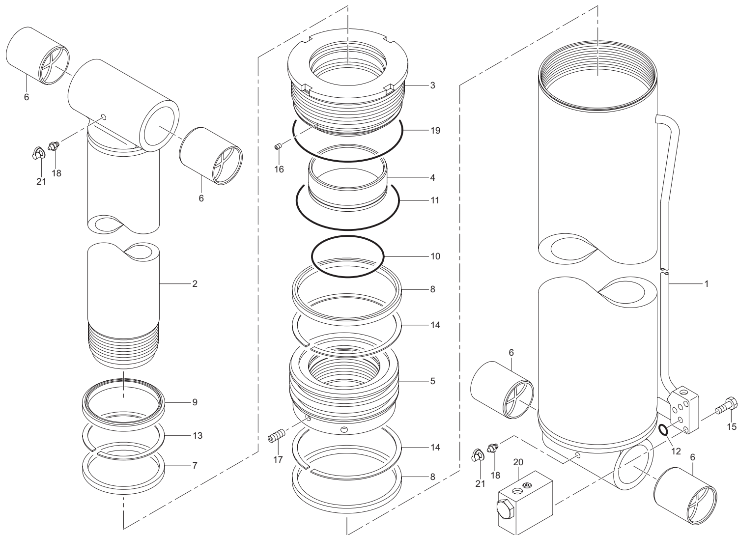
デリックシリンダ組立 (URV500-1-GO 系) Fig. 11-1 DERRICK CYLINDER ASS'Y (URV500-1-GO series)
