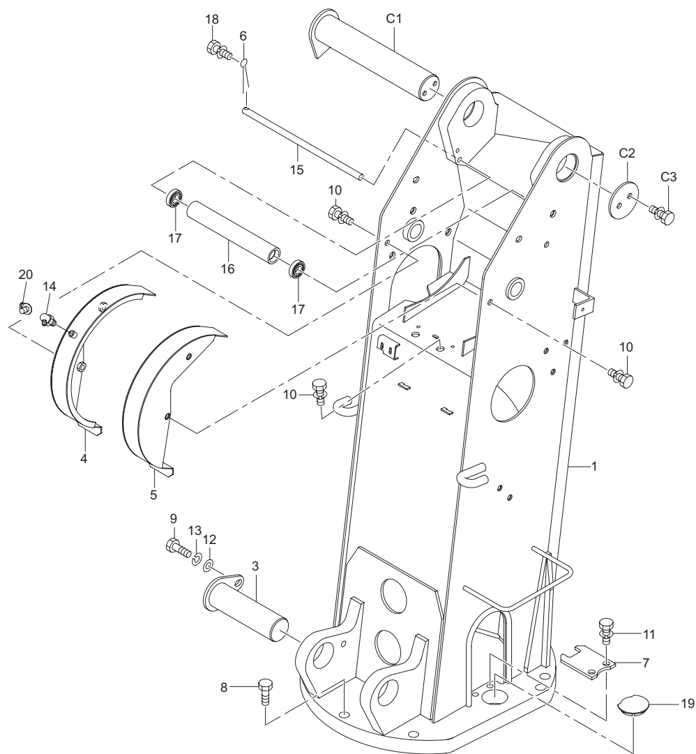
コラム組立 (URV500-1-GO 系) Fig.7-1 COLUMN ASS'Y(URV500-1-GO series)
