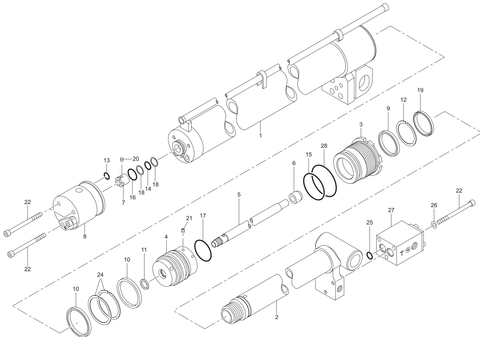
テレシリンダ (1) 組立 (URV503-1-GO) Fig. 2-1 TELESCOPE CYLINDER(1) ASS'Y(URV503-1-GO)
