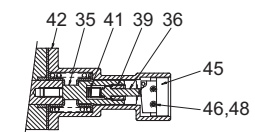
C-C 断面 SECTION C-C
