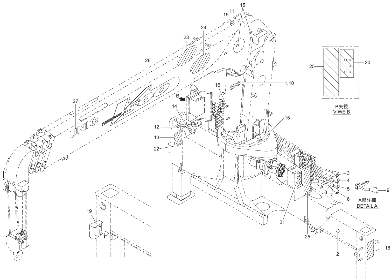
銘板 (URV500-1-GO 系) Fig. 16-2 NAME PLATE (URV500-1-GO series)
