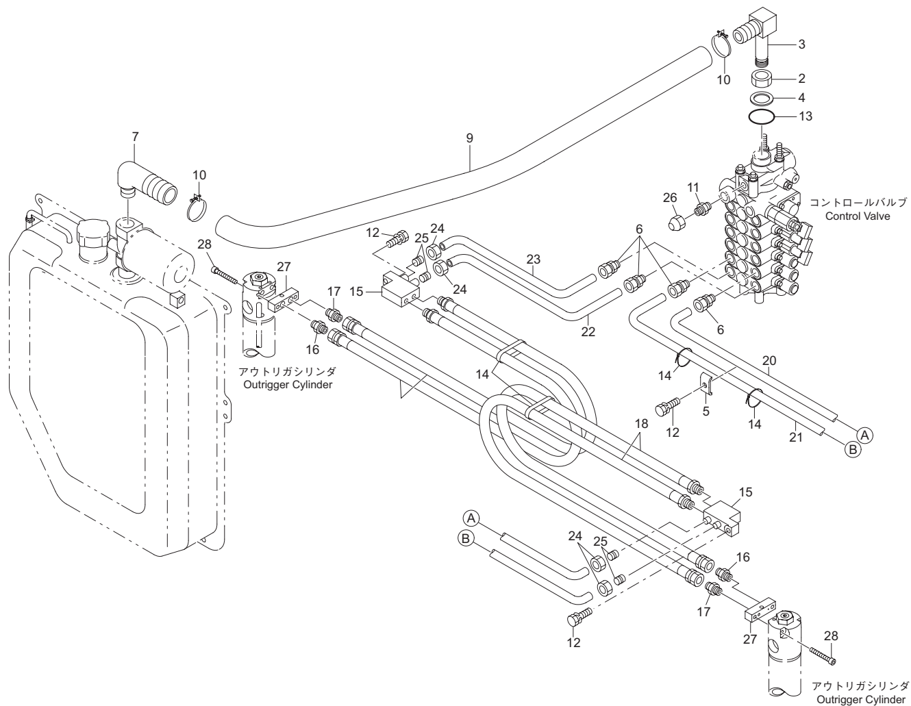
パイピング (アウトリガ) (URV370-GO 系) Fig. 6-2-5 PIPING(Outrigger)(URV370-GO series)
