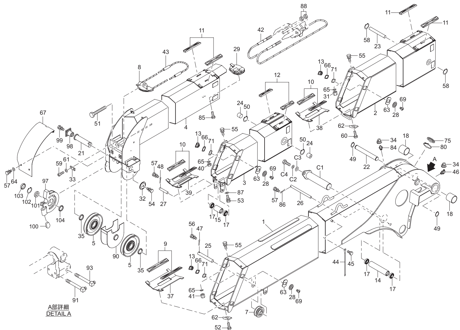
4 段ブーム組立 (URV374-GO) Fig.1-8 4-section BOOM ASS'Y(URV374-GO)
