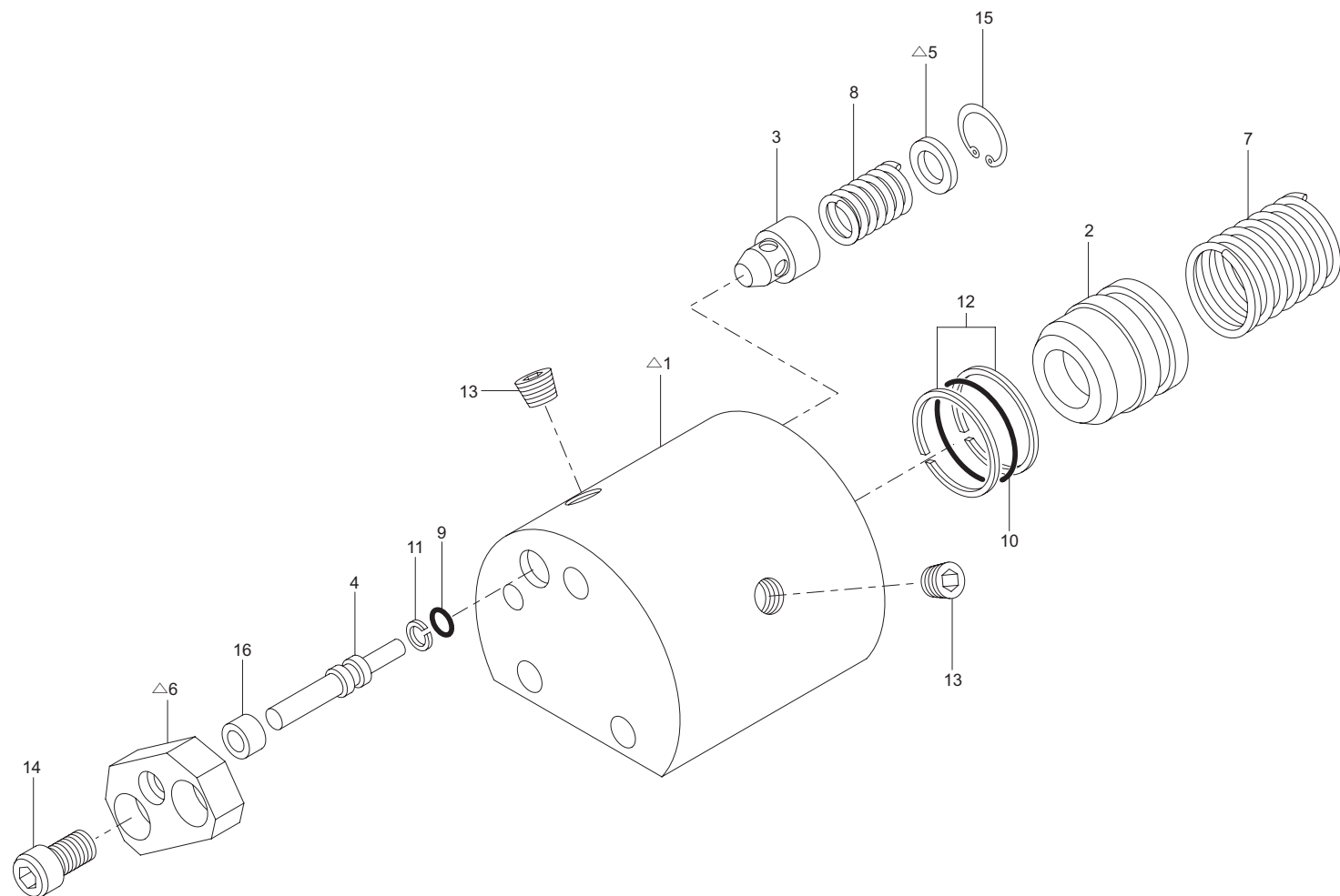
切換バルブ ASS'Y(URV374-GO) Fig. 2-4-1 SELECTOR VALVE ASS'Y(URV374-GO)
