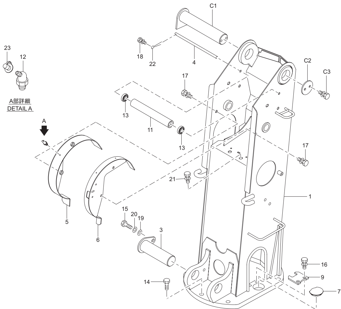
コラム組立 (URV370-GO 系) Fig.7-1 COLUMN ASS'Y(URV370-GO series)
