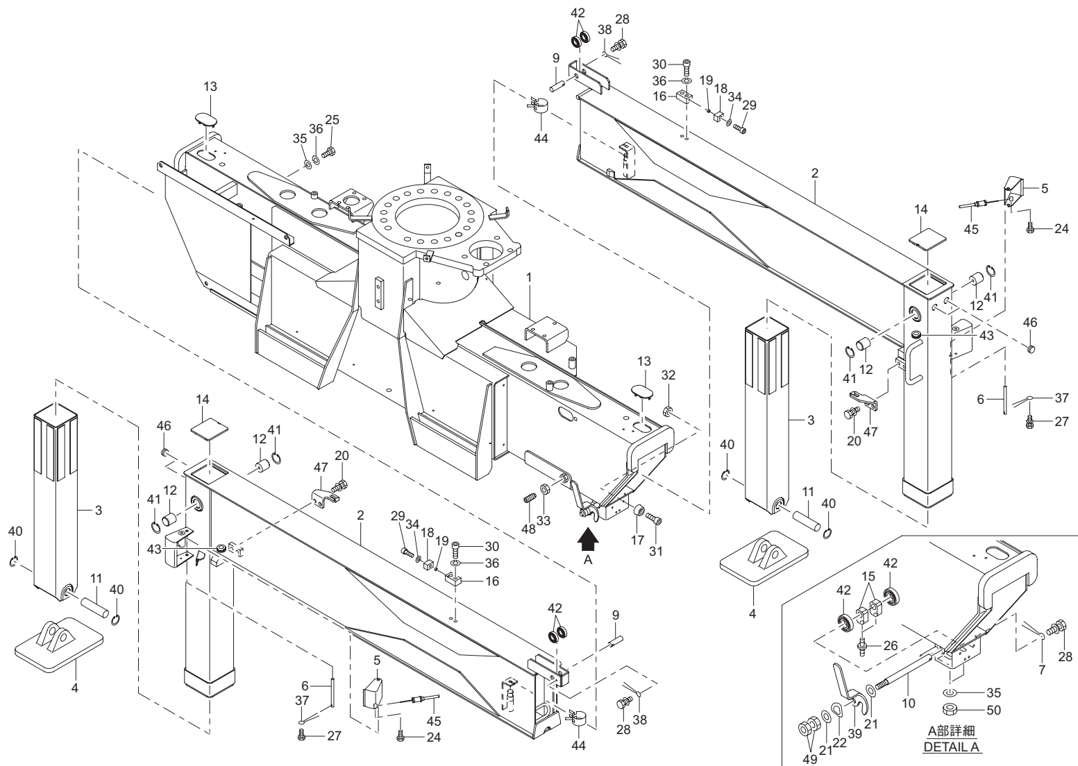
ベース組立 (URV370-GO 系) Fig. 8-1 BASE ASS'Y (URV370-GO series)
