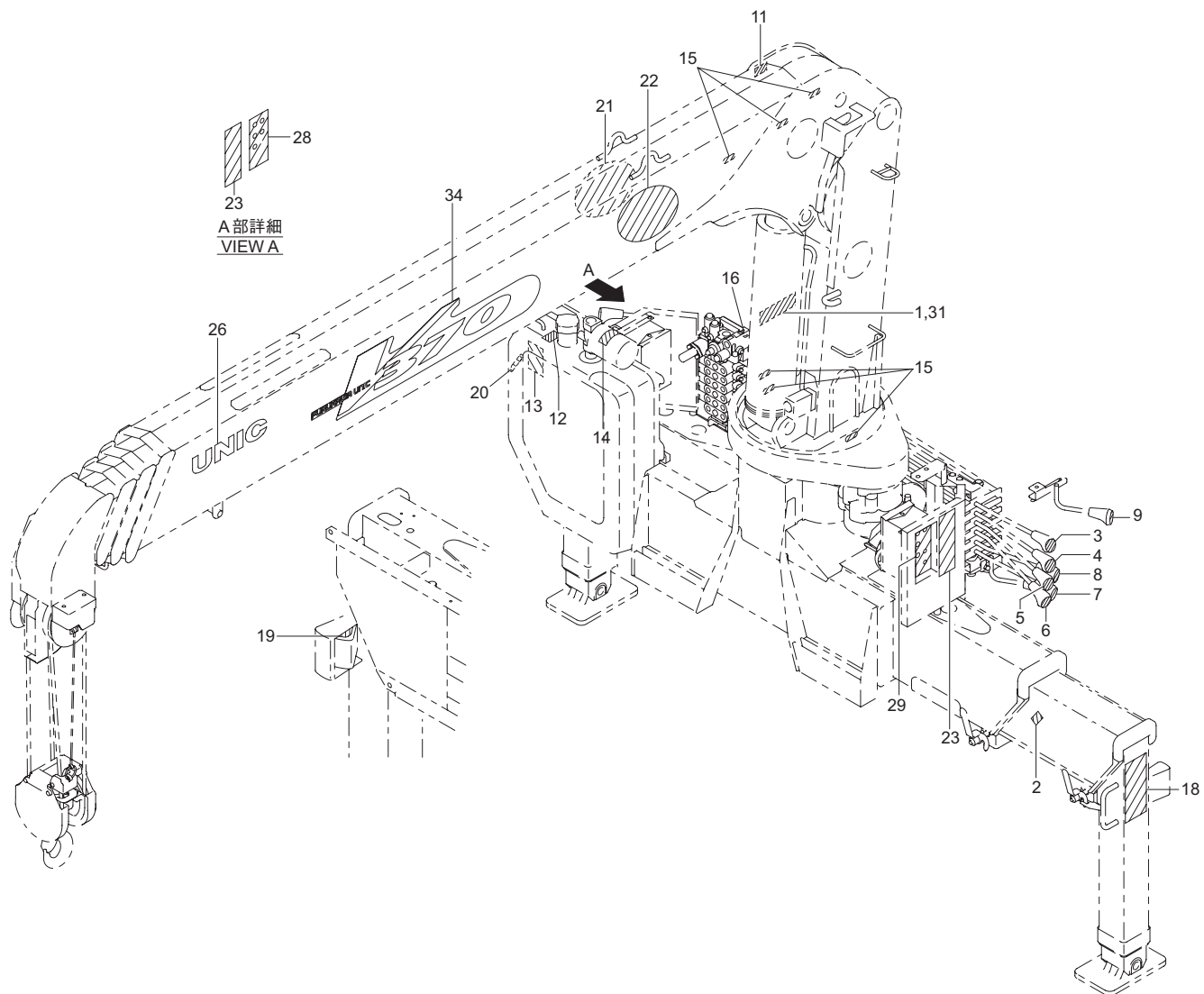
銘板 (URV370-GO 系) Fig. 16-2 NAME PLATE(URV370-GO series)
