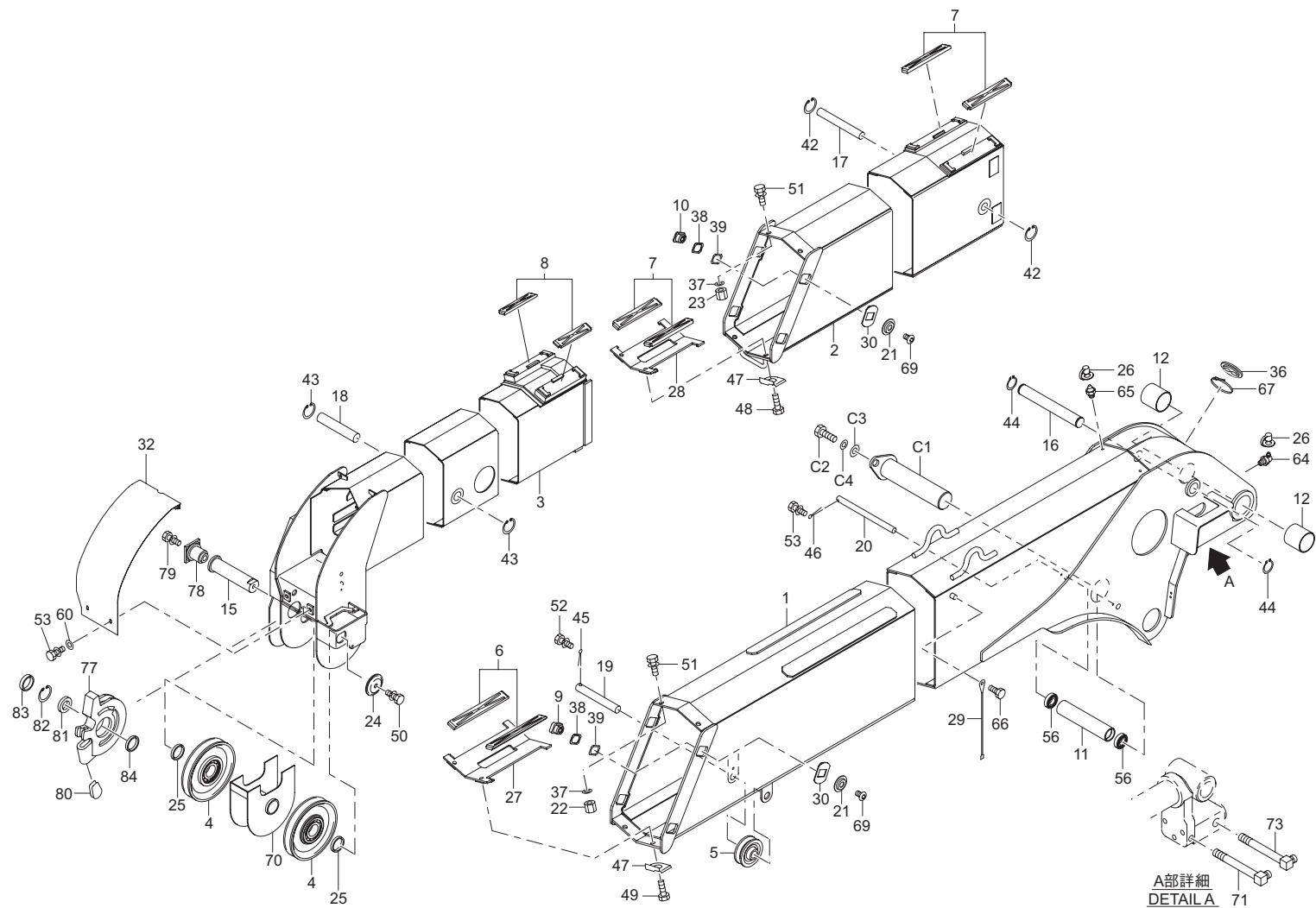
3 段ブーム組立 (URV373-GO) Fig.1-5 3-section BOOM ASS'Y(URV373-GO)
