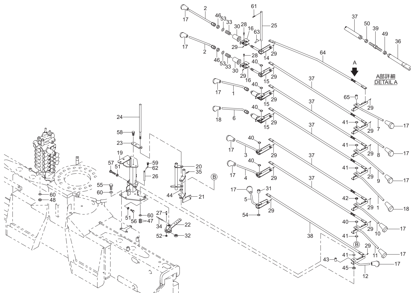
コントロール組立 (URV370-GO 系) Fig. 14-2 CONTROL ASS'Y (URV370-GO series)
