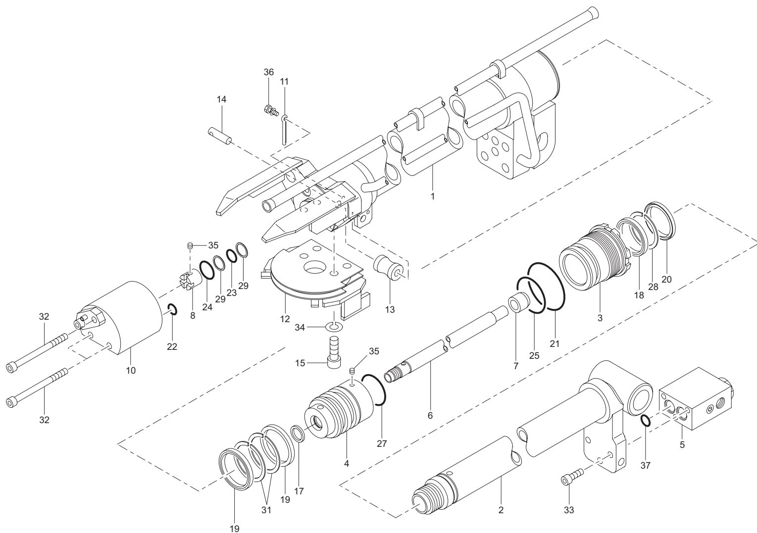
テレシリンダ (1) 組立 (URV374-GO) Fig. 2-4 TELESCOPE CYLINDER(1) ASS'Y(URV374-GO)
