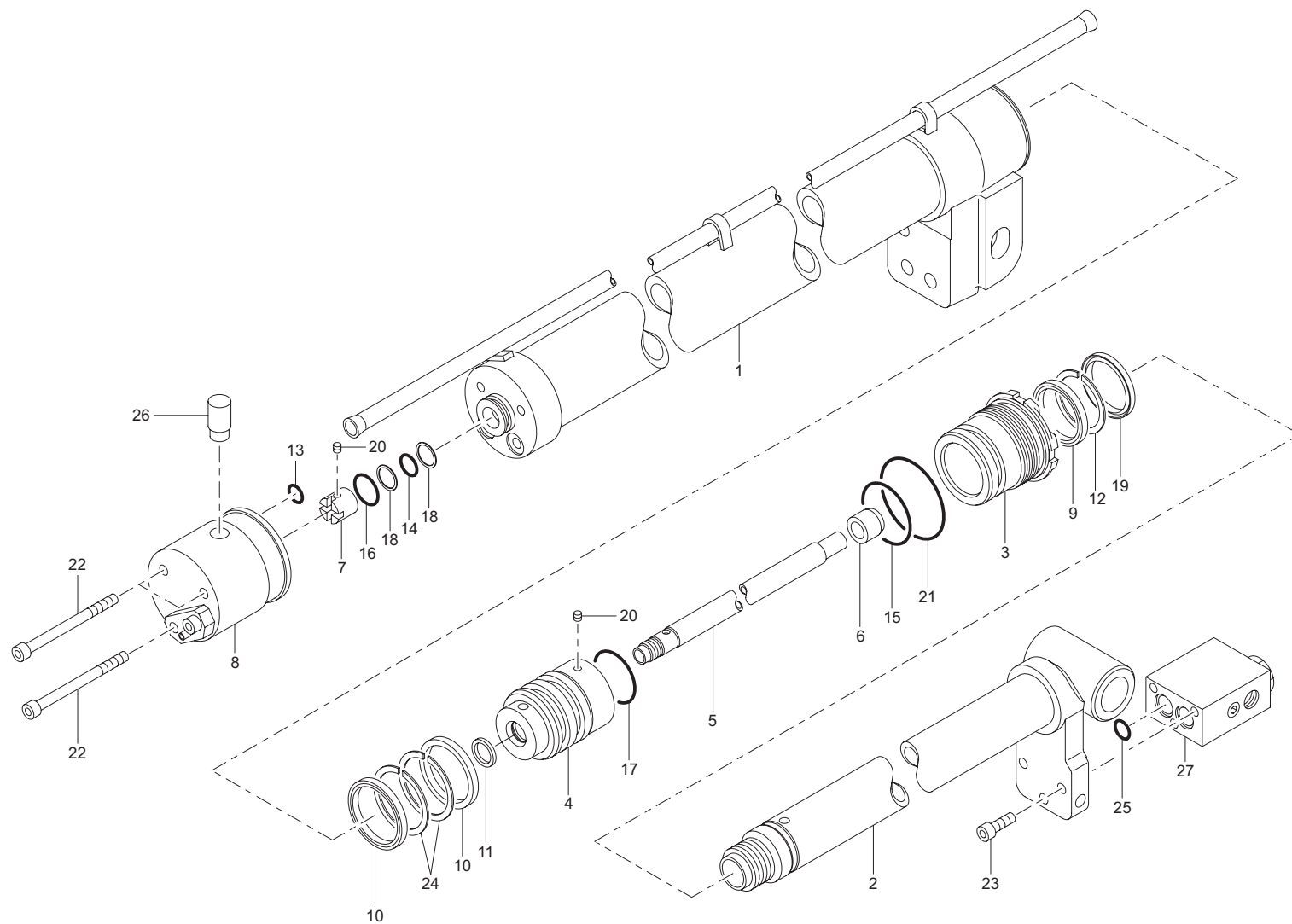
テレシリンダ (1) 組立 (URV373-GO) Fig. 2-2 TELESCOPE CYLINDER(1) ASS'Y(URV373-GO)
