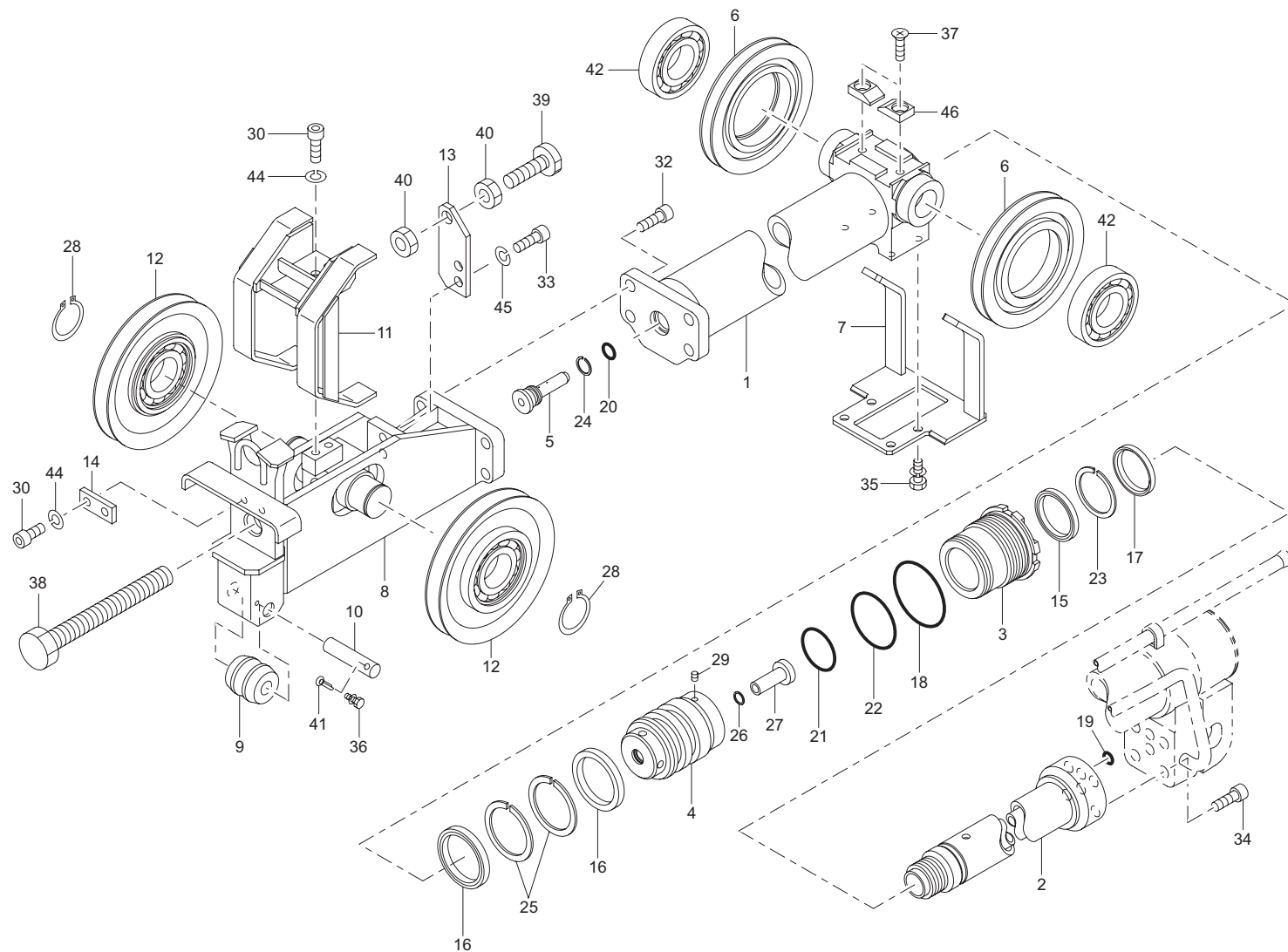
テレシリンダ (2) 組立 (URV374-GO) Fig. 2-5 TELESCOPE CYLINDER(2) ASS'Y(URV374-GO)
