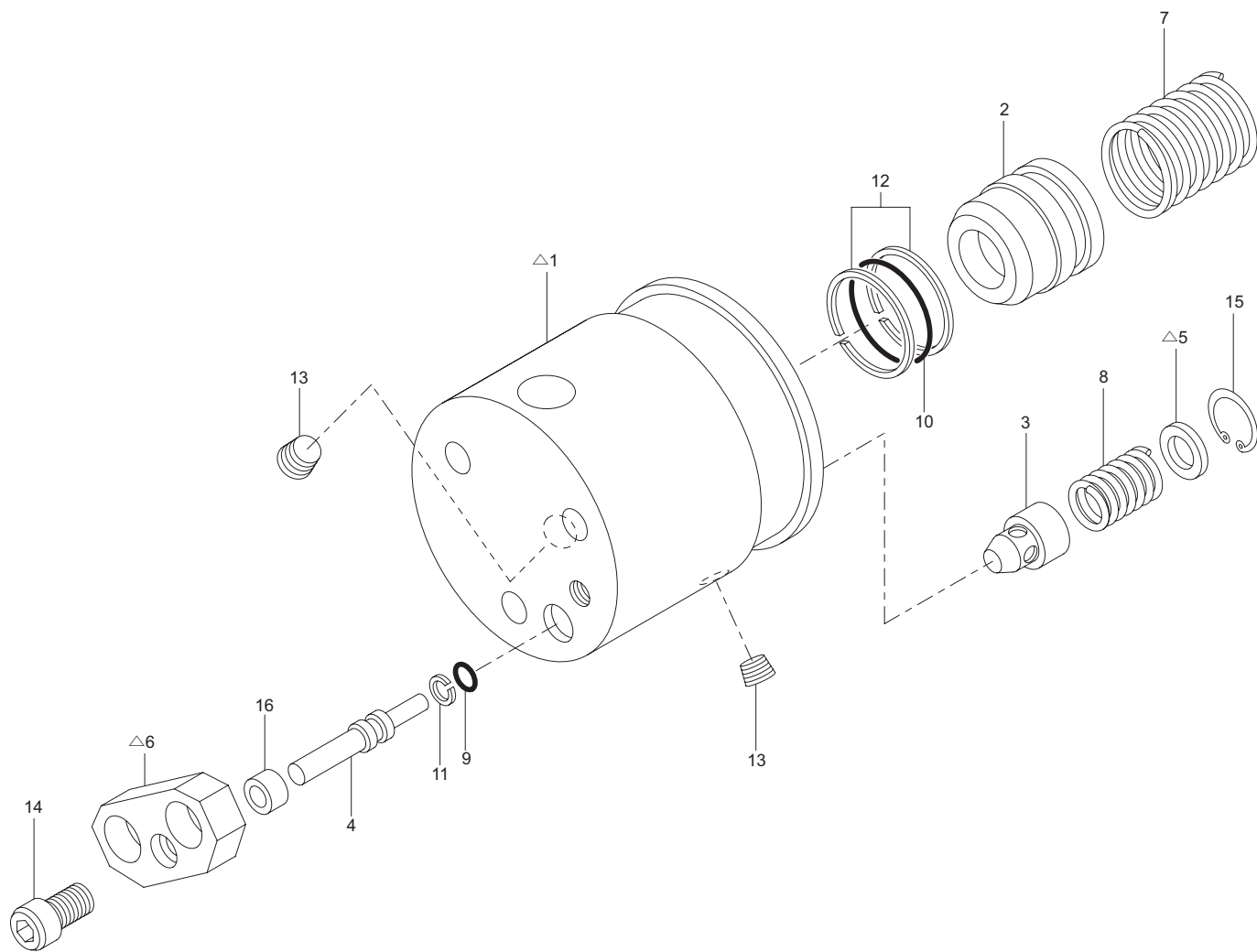
切換バルブ ASS'Y(URV373-GO) Fig. 2-2-1 SELECTOR VALVE ASS'Y(URV373-GO)
