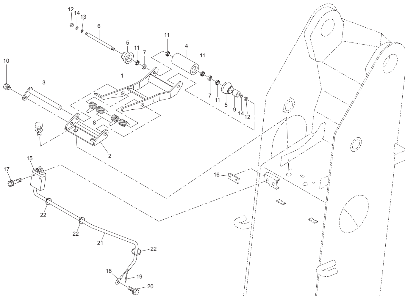
ワイヤロープ押えローラ装置組立 (URV370-GO 系) Fig. 19-1 WIRE ROPE CLAMPING ROLLER DEVICE ASS'Y (URV370-GO series)
