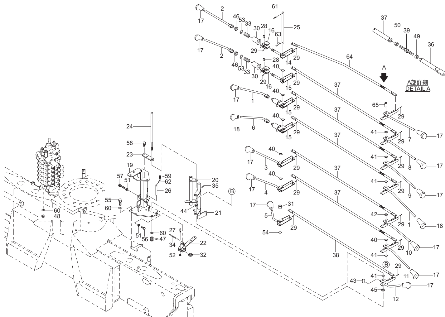
Fig. 14-2 コントロール組立 (URV370-GO 系) CONTROL ASS'Y (URV370-GO series)
