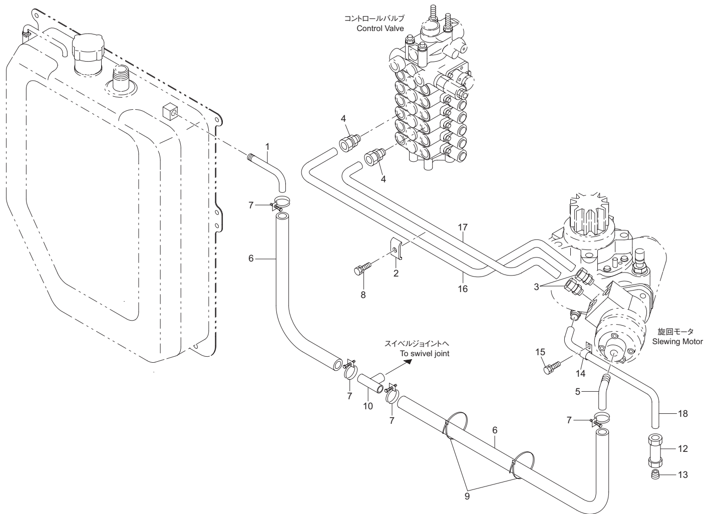
パイピング (旋回モータ) (URV370-GO 系) Fig. 6-2-4 PIPING(Slewing motor)(URV370-GO series)
