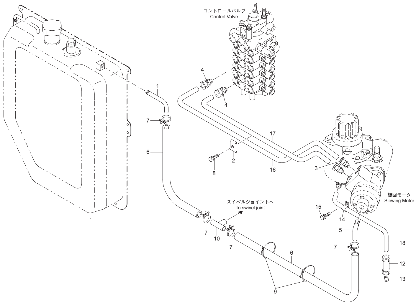
パイピング (旋回モータ) (URV340-GO 系) Fig. 6-2-4 PIPING(Slewing motor)(URV340-GO series)
