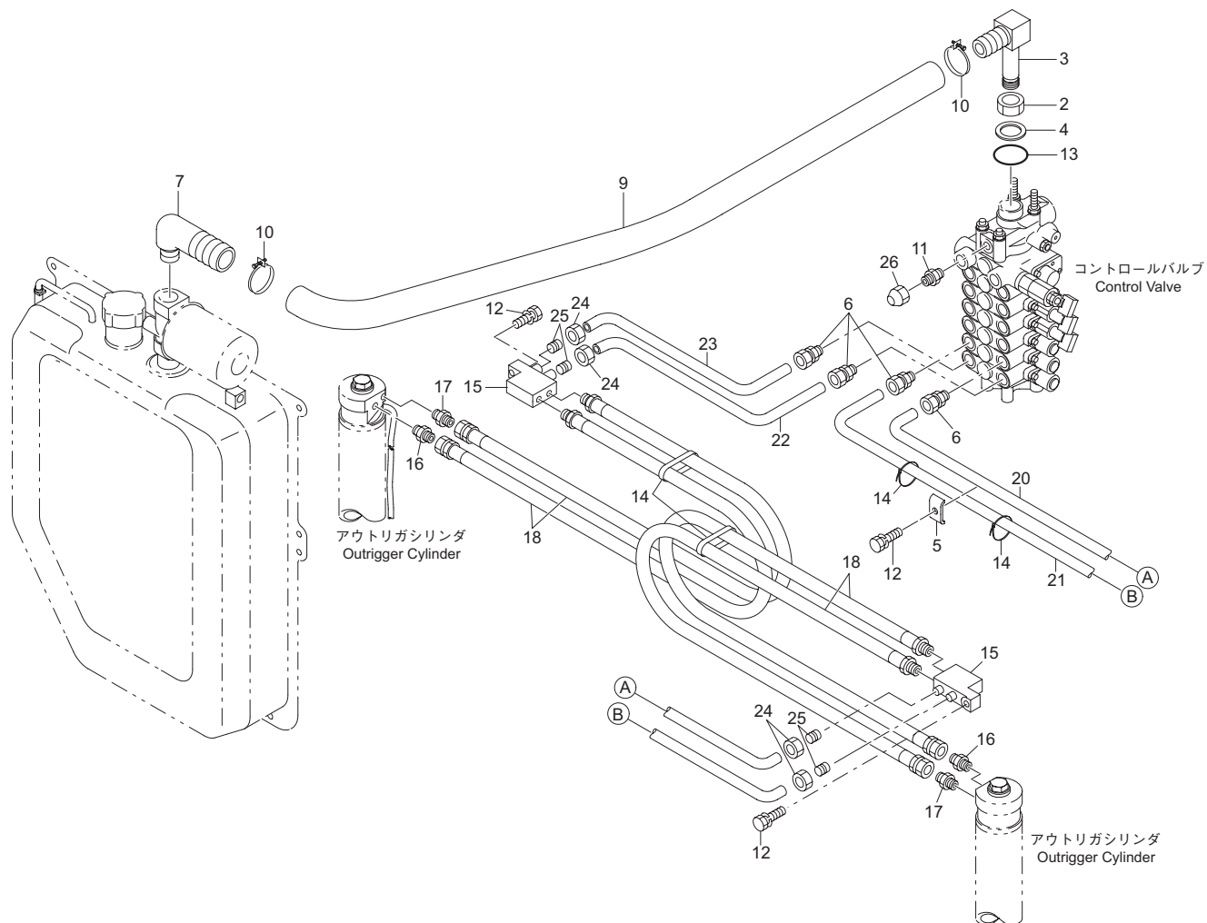
パイピング (アウトリガ) (URV340-GO 系) Fig. 6-2-5 PIPING(Outrigger) (URV340-GO series)
