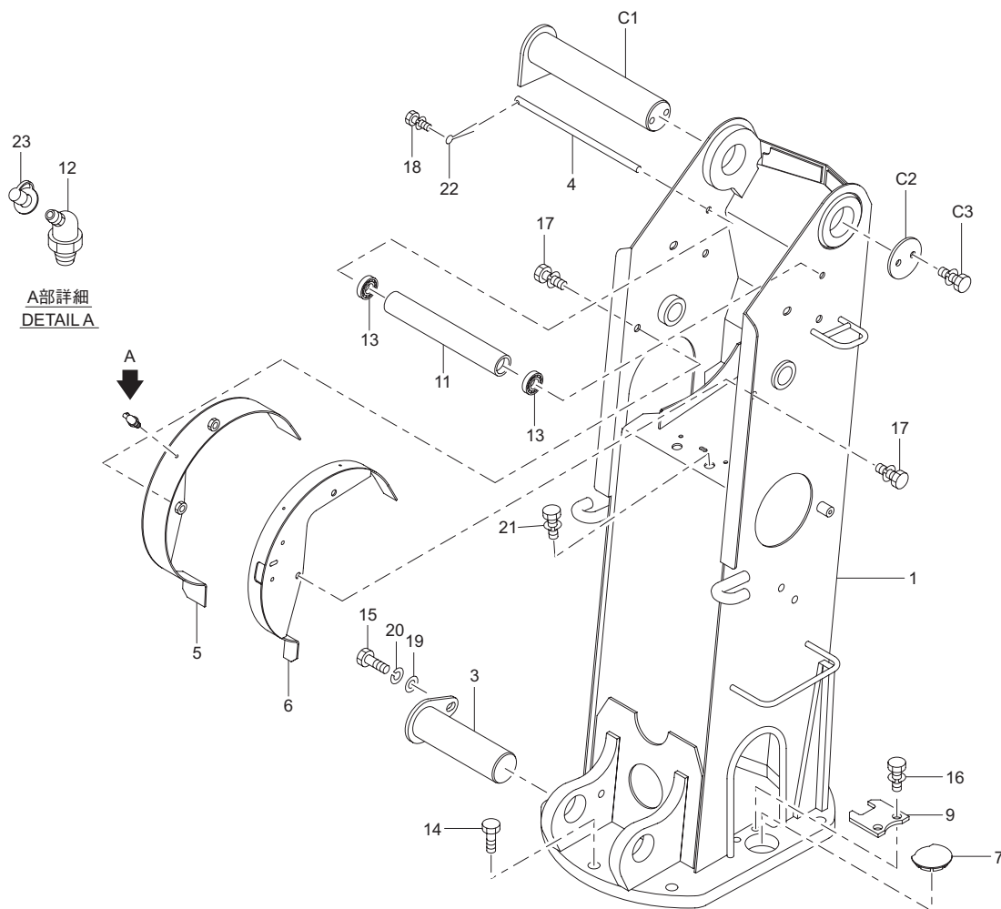
Fig.7-1 コラム組立 (URV340-GO 系) COLUMN ASS'Y (URV340-GO series)
