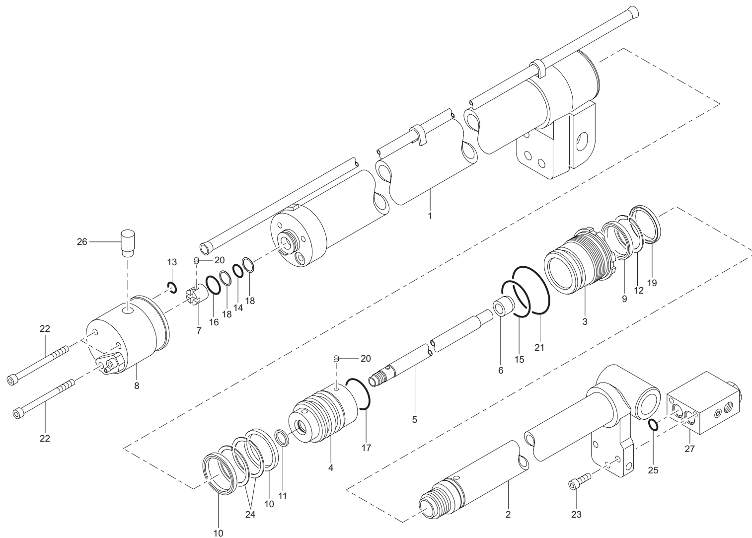
テレシリンダ (1) 組立 (URV343-GO) Fig. 2-2 TELESCOPE CYLINDER(1) ASS'Y(URV343-GO)
