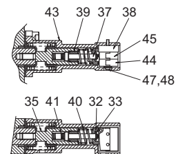
E 部詳細 DETAIL E
