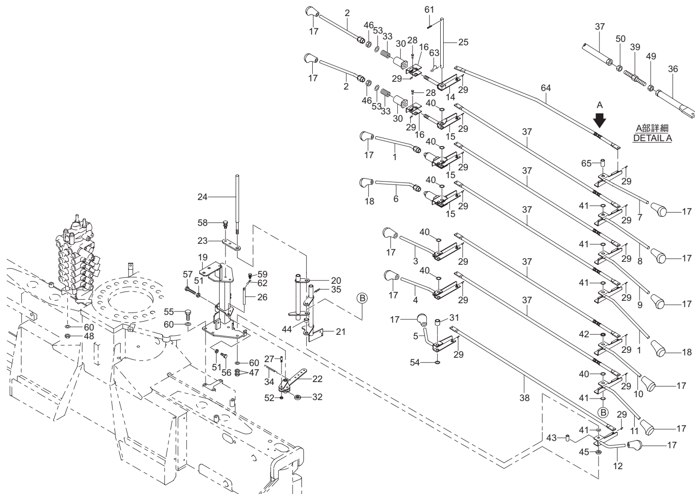
コントロール組立 (URV340-GO 系) Fig. 14-2 CONTROL ASS'Y (URV340-GO series)
