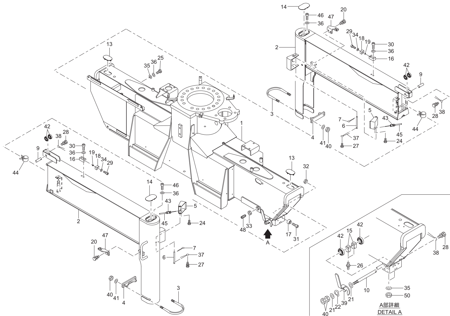
ベース組立 (URV340-GO 系) Fig. 8-1 BASE ASS'Y (URV340-GO series)
