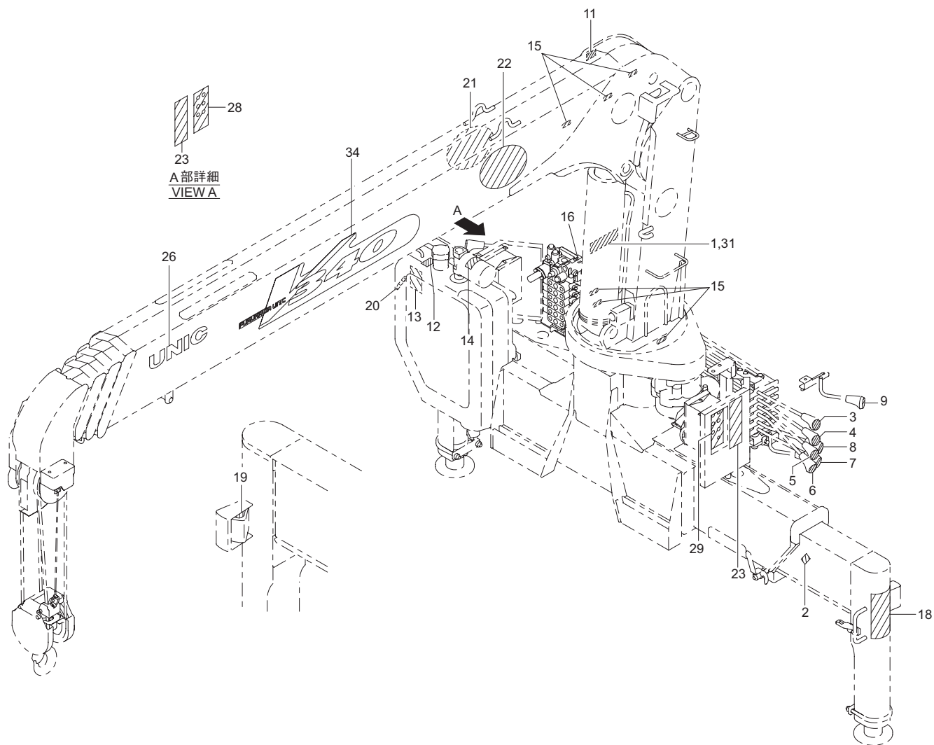
銘板 (URV340-GO 系) Fig. 16-2 NAME PLATE(URV340-GO series)
