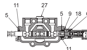
A-A 断面 SECTION A-A
