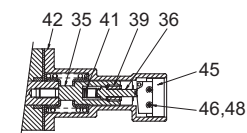
C-C 断面 SECTION C-C
