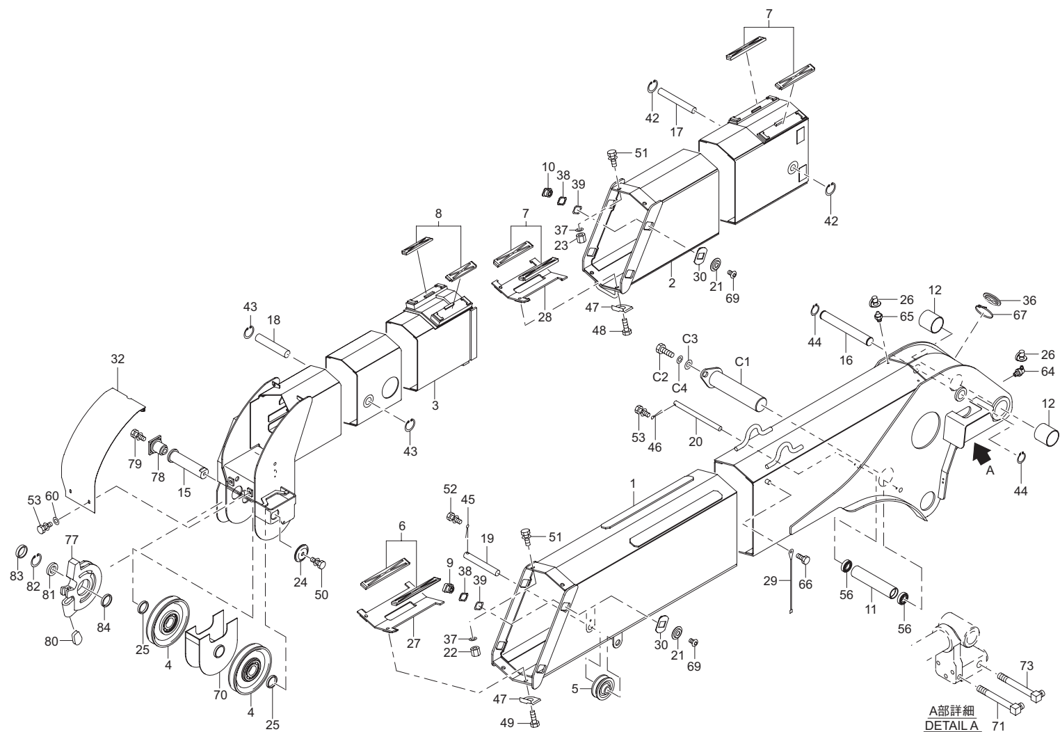
3 段ブーム組立 (URV343-GO) Fig.1-5 3-section BOOM ASS'Y(URV343-GO)
