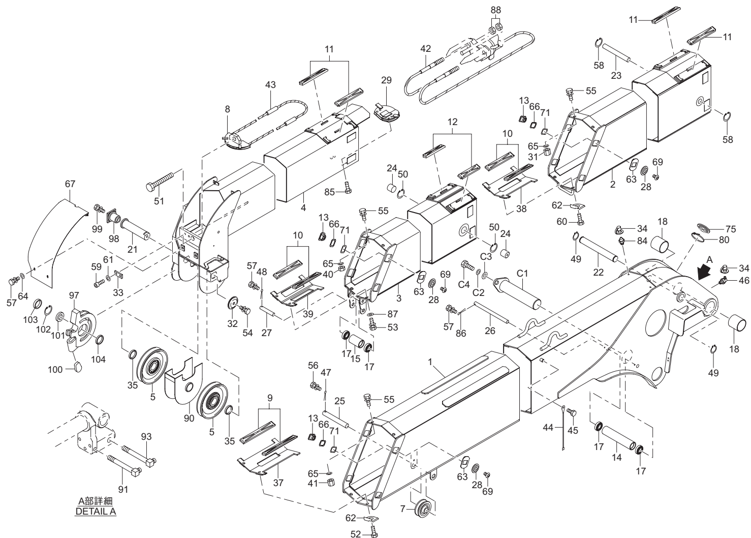
4 段ブーム組立 (URV344-GO) Fig.1-8 4-section BOOM ASS'Y(URV344-GO)
