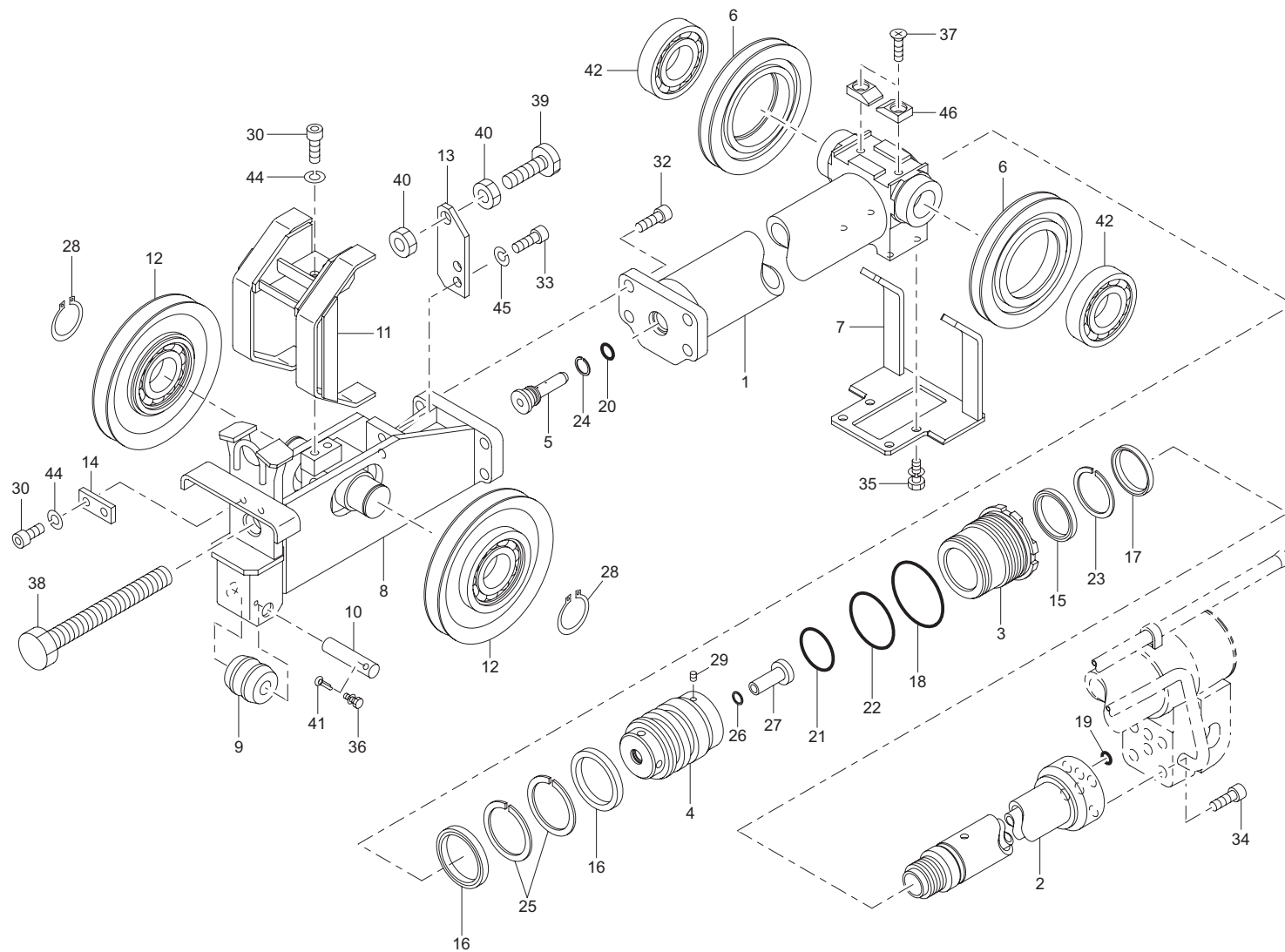
テレシリンダ (2) 組立 (URV344-GO) Fig. 2-5 TELESCOPE CYLINDER(2) ASS'Y(URV344-GO)
