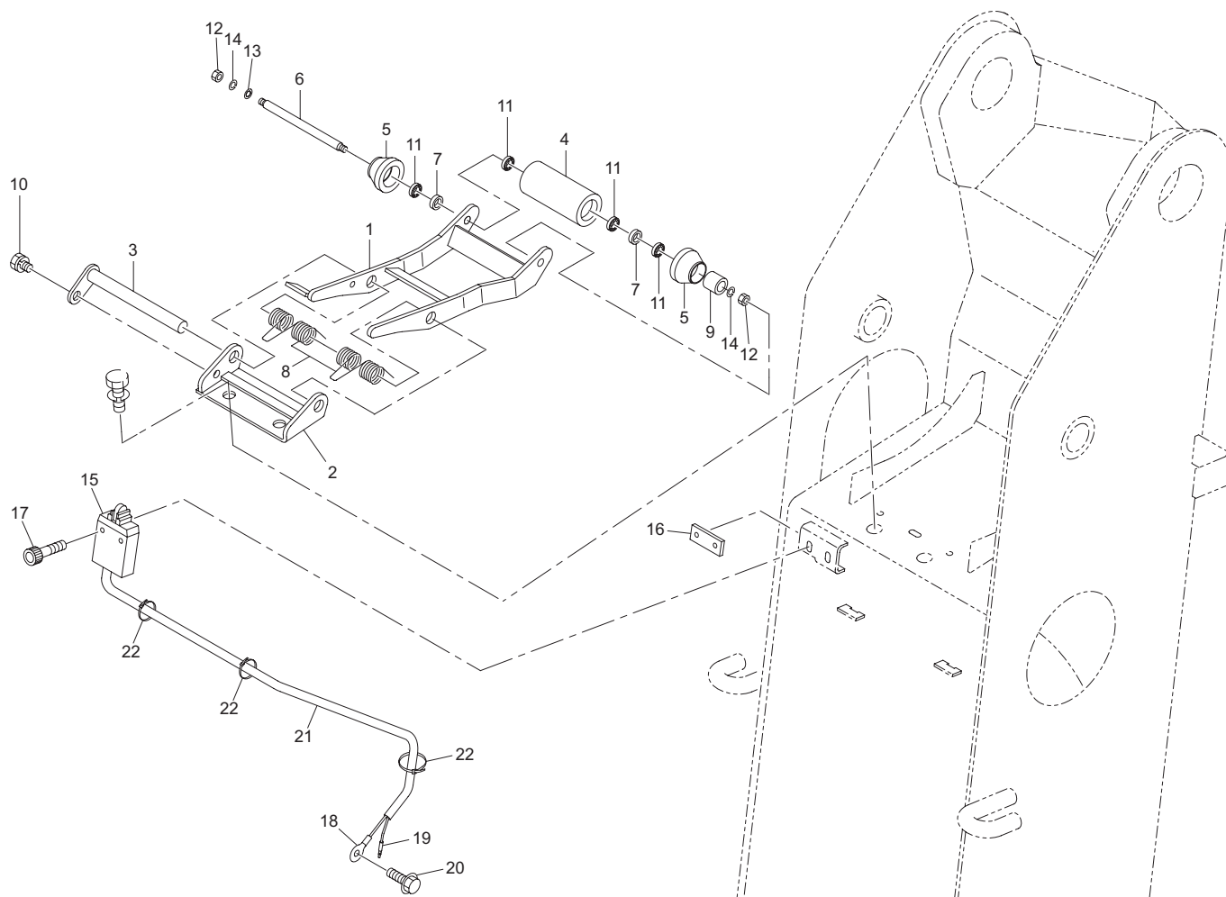
ワイヤロープ押えローラ装置組立 (URV340-GO 系) Fig. 19-1 WIRE ROPE CLAMPING ROLLER DEVICE ASS'Y (URV340-GO series)
