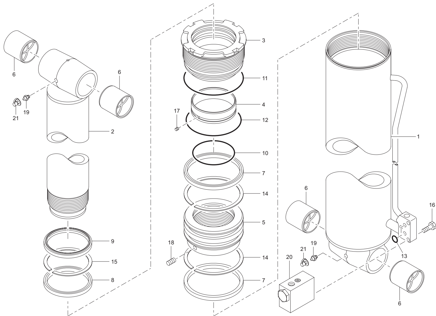
Fig.11-1 デリックシリンダ組立 (URV340-GO 系) DERRICK CYLINDER ASS'Y (URV340-GO series)
