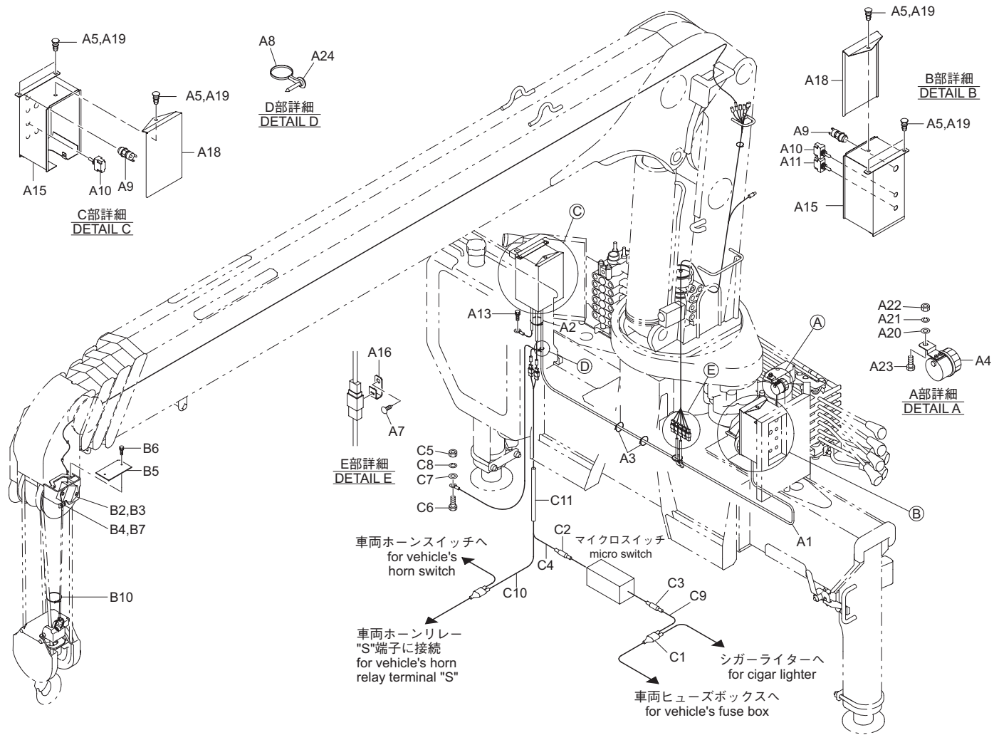
警報装置組立 (URV340-GO 系) Fig. 4-2 ALARM DEVICE ASS'Y (URV340-GO series)
